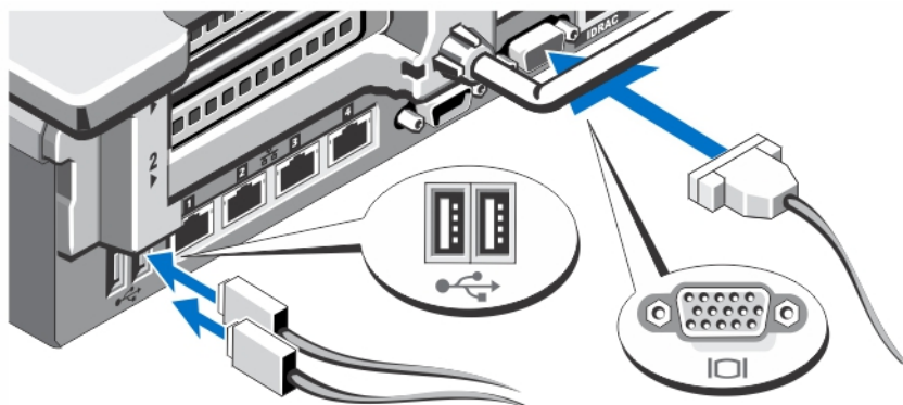
Ilustración 2. Opcional: conexión del teclado, el mouse y el monitor
